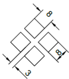
Perforacja rombu
