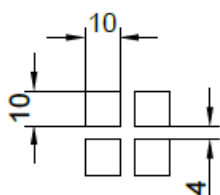
Perforacja kwadratu
